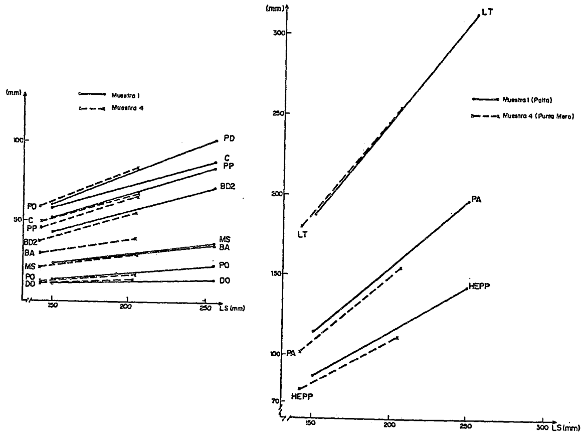
Fig 6. Relación entre la longitud estandar (LS) y otros caracteres para Cynoscion analis (Muestra 1) y Cynoscion altipinnis (Muestra 4) (PD= long. pre-dorsal; C= long. cabeza; PP= long. pre-pectoral; BD2= long. base segunda dorsal; BA= long. base anal; PO= long. pre-orbital; DO= diámetro orbital; LT= long. total; PA= long. pre-anal; HEPP= long. hocico - extremo posterior de la pectoral)
