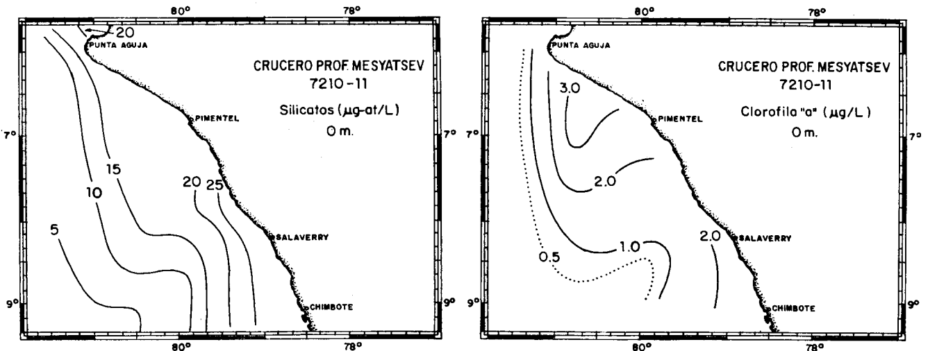
Fig. 8b Distribución de silicatos y clorofila "a" en la superficie del mar
