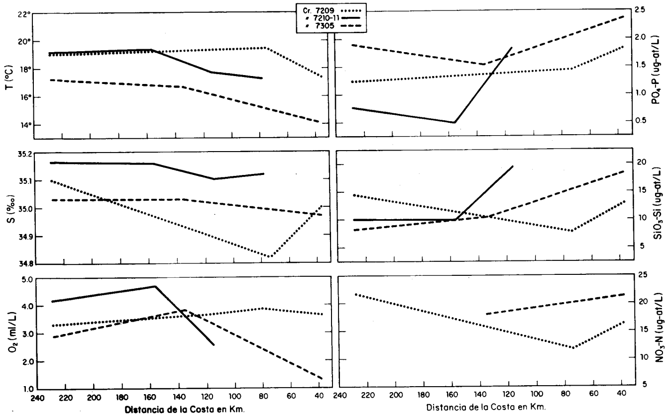
Fig. 28 Variaciones de la temperatura, salinidad, oxígeno disuelto, nitratos, silicatos y fosfatos promedios en la columna de agua de 0 - 50 m con la distancia de la costa
