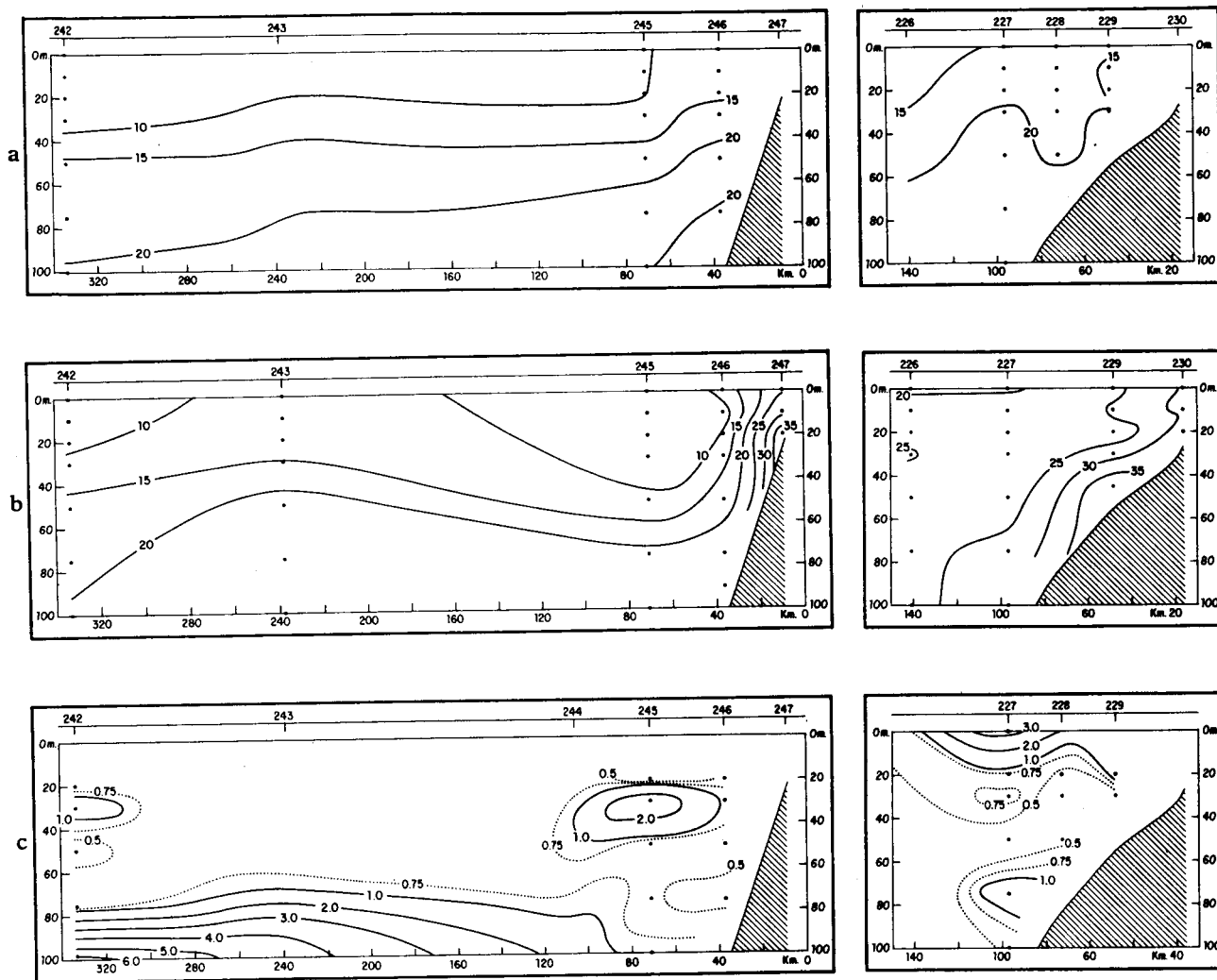
Fig. 7b Chimbote Sección de: a) nitratos ( \mu\text{g-at/L} ), b) silicatos ( \mu\text{g-at/L} ), c) feo- pigmentos ( \mu\text{g/L} ) frente a Chimbote durante el invierno del 1972 (Cr. 7209)
