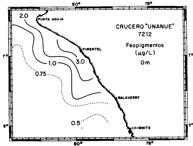
Fig. 12b Distribución de silicatos, clorofila "a" y feopigmentos en la superficie del mar
