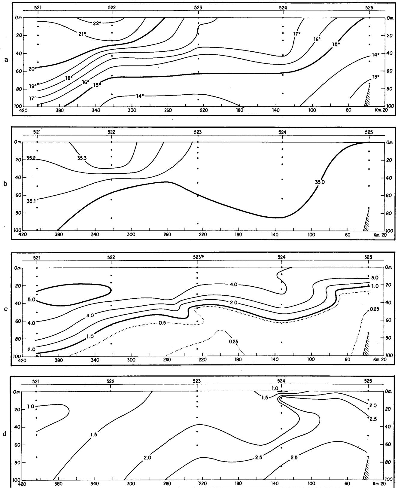
Fig. 21a Chimbote - Pimentel Sección de: a) temperatura (°C), b) salinidad, c) oxígeno disuelto, d) fosfatos, frente a Chimbote y Pimentel durante otoño de 1973 (Cr. 7305)
