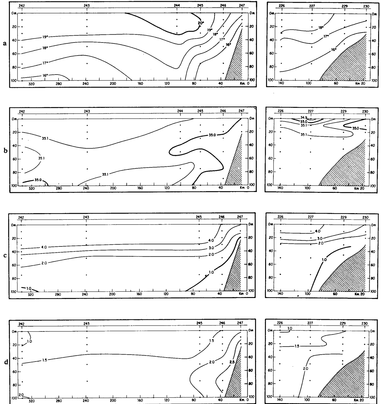
Fig. 7a Chimbote - Pimentel Sección de: a) temperatura (°C), b) salinidad (‰), oxígeno disuelto (ml/L y fosfatos (µg-at/L) durante el invierno de 1972 (Cr. 7209)
