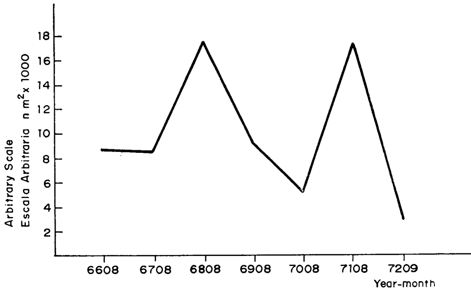
Figura 5.—Estimado de abundancia del stock por las Eureka de Verano (Areas de densidad ponderadas con valores de calibración del eco-integrador y ajustadas para la cobertura de latitudes en las prospecciones).
