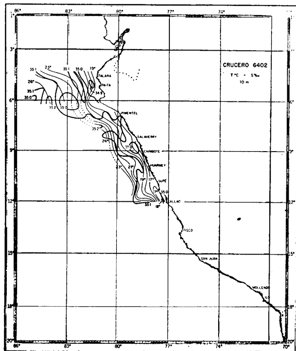
Figura 2a. Distribución de la temperatura (—) y la salinidad (---) al nivel de 10 m. durante el Verano de 1964.
