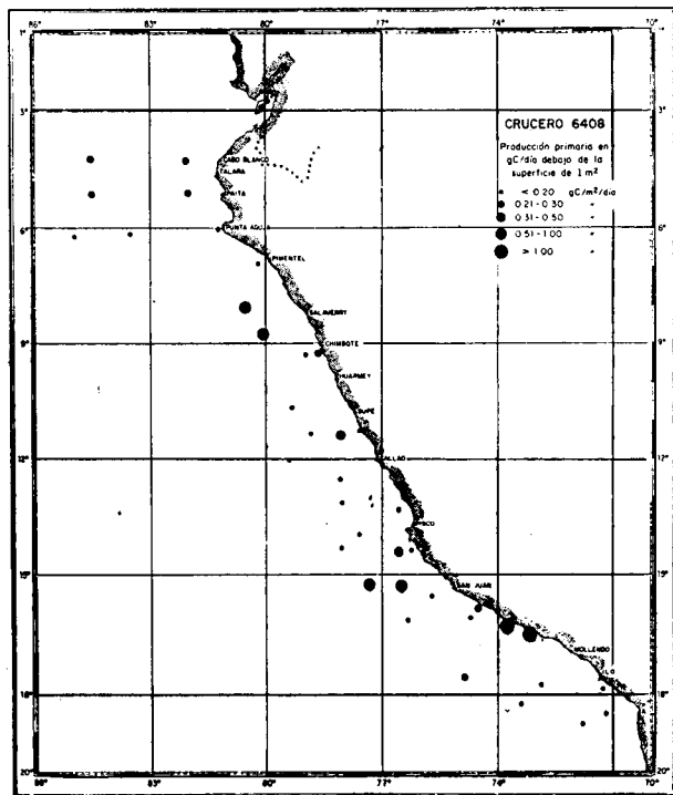
Figura 3c. Distribución de la Producción Primaria en la columna de agua durante el Invierno de 1964.
