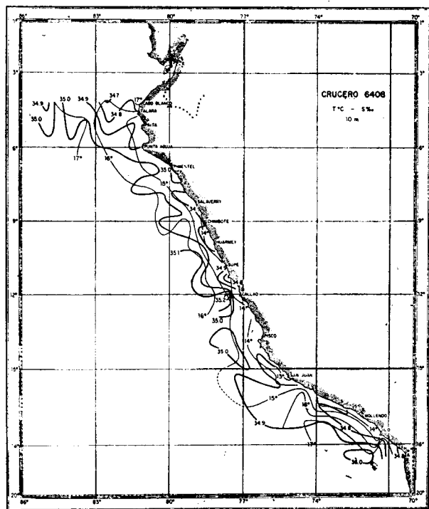
Figura 2c. Distribución de la temperatura (—) y la salinidad (---) al nivel de 10 m. durante el Invierno de 1964.
