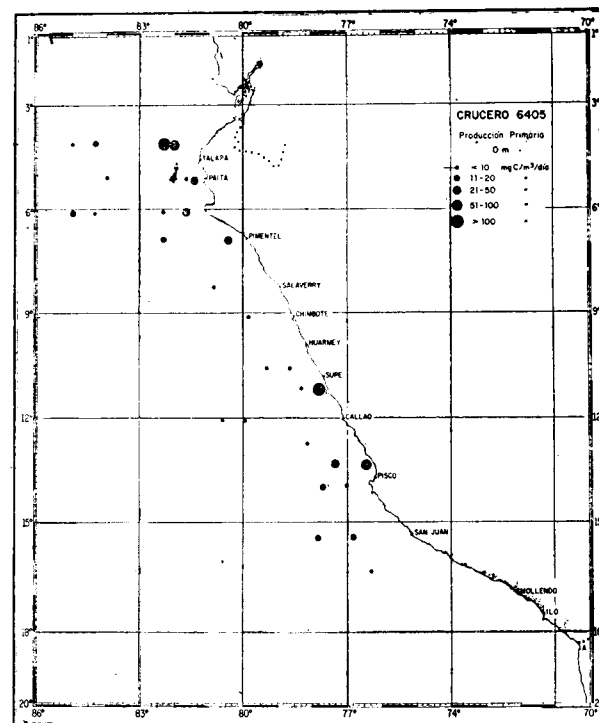
Figura 6b. Distribución de la Producción Primaria en superficie, durante el Otoño de 1964.
