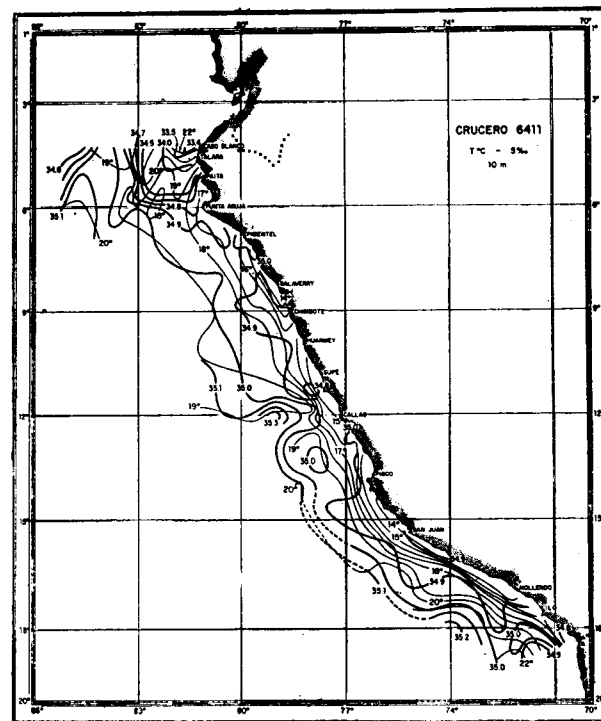
Figura 2d. Distribución de la temperatura (—) y la salinidad (---) al nivel de 10 m. durante la Primavera de 1964.
