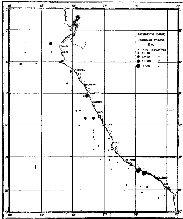
Figura 6c. Distribución de la Producción Primaria en superficie, durante el Invierno de 1964.
