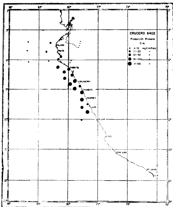
Figura 6a. Distribución de la Producción Primaria en superficie, durante el Verano de 1964.
