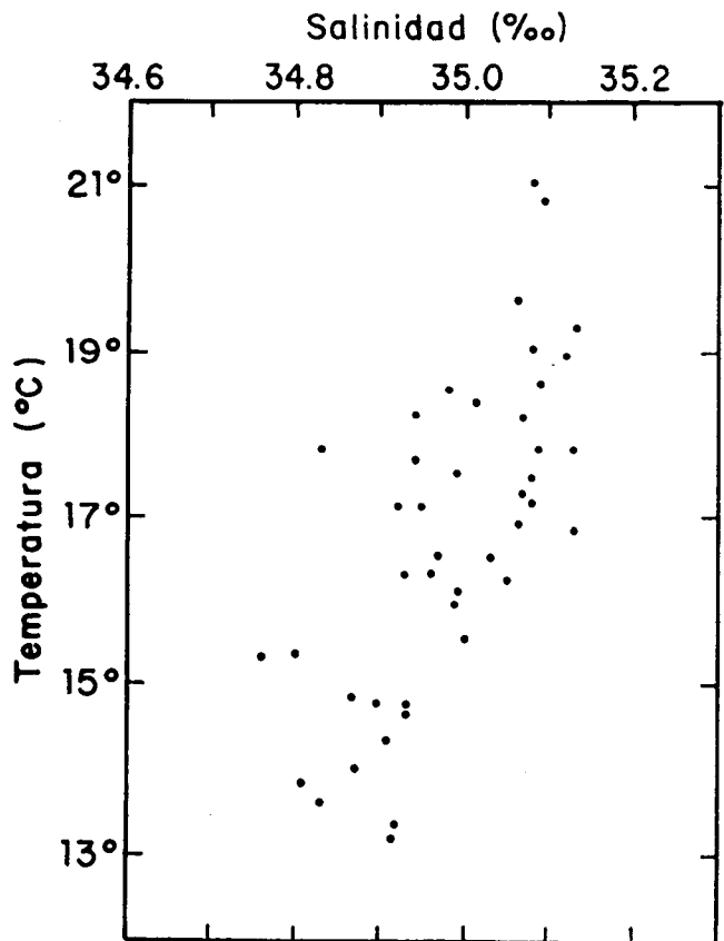
Figura 4 Diagrama Temperatura-Salinidad con valores promedios para la capa de 0-20 m., correspondiente a estaciones con valores mayores de 0.35 \text{ gr C/m}^2/\text{día} .
