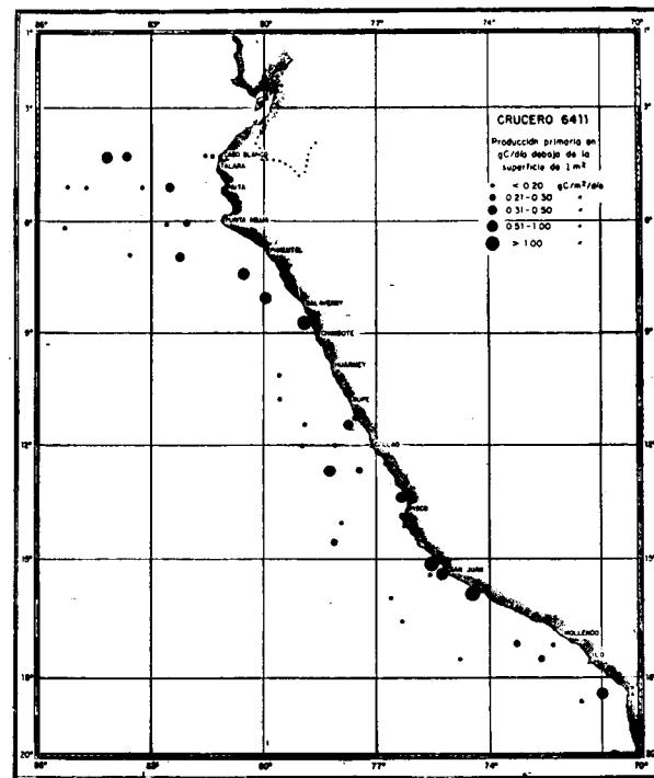
Figura 3d. Distribución de la Producción Primaria en la columna de agua durante la Primavera de 1964.
