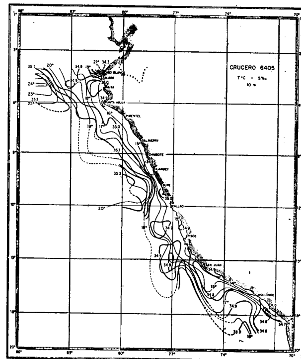
Figura 2b. Distribución de la temperatura (—) y la salinidad (---) al nivel de 10 m. durante el Otoño de 1964.
