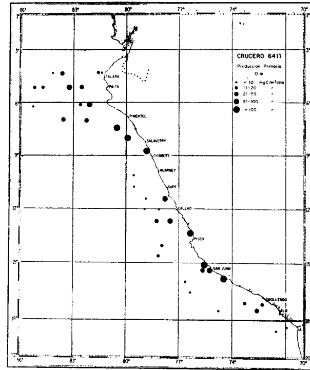
Figura 6d. Distribución de la Producción Primaria en superficie, durante la Primavera de 1964.
