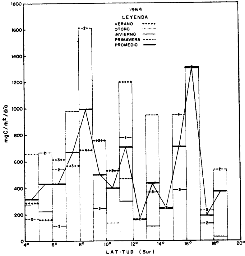
Figura 7 Variación latitudinal de la Producción Primaria en la columna de agua, durante las cuatro estaciones del año 1964.
