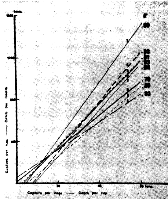
Figura 8.— Regresiones lineales de captura mensual sobre captura por viaje con captura y los coeficientes de correlación. Los números se refieren a los diferentes grupos de datos (ver Tabla 13). Figure 8.— Linear regressions of monthly catch on catch per trip with catch and the correlation coefficients. Numbers refer to different groups of data (see Table 13).
