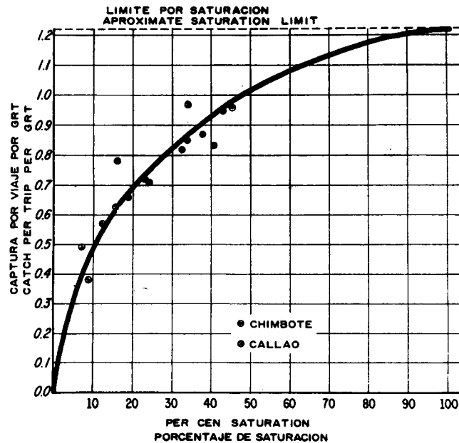
Figura 14.— Ploteo de la ocurrencia promedio de saturación contra captura promedio por viaje por GRT. Curva trazada al ojo.
