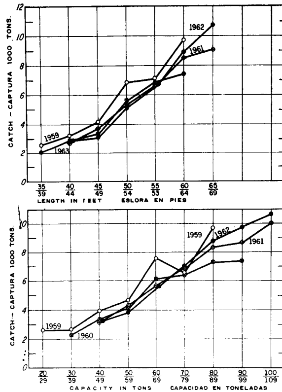
Figura 7.— Relación entre captura media anual de las embarcaciones seleccionadas y el tamaño de la embarcación. Todos los puertos tomados en conjunto, 1959-1962. Figure 7.— Relation between mean annual catch of selected vessels and vessel size. All ports taken together, 1959-1962.
