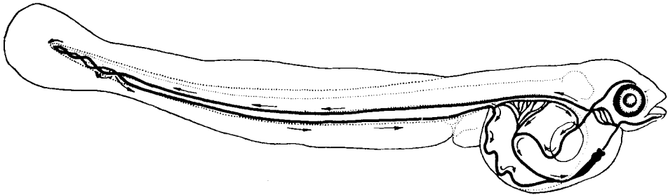
Fig. 1.— Esquema de una larva recién eclosionada donde se aprecian los detalles de la circulación.
